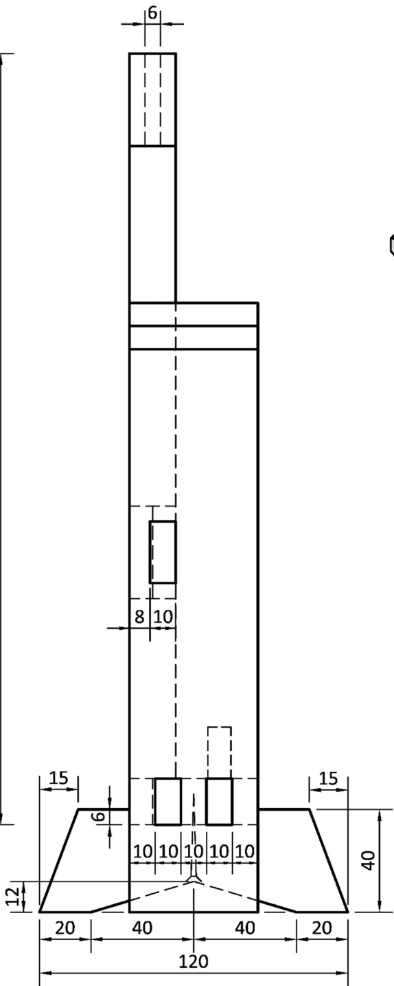
End View/Taobhchló
